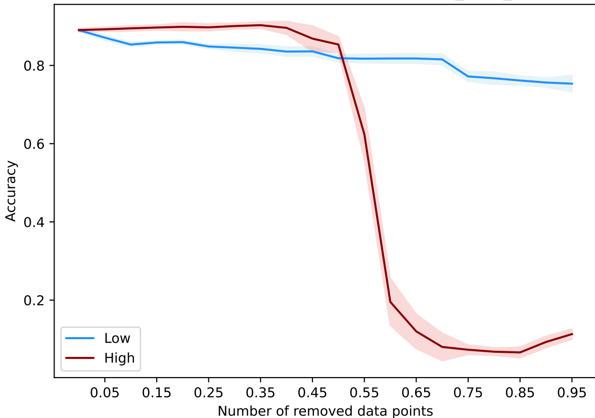
DataOob(1000, epochs=15) - nomaoworst_class_acc
